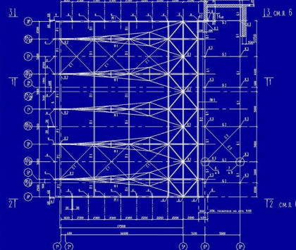
СХЕМА МЕТАЛЛОКОНСТРУКЦИЙ ПОКРЫТИЯ
