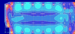
цветовое изображение моментов в расчётных схемах фундаментной плиты и встраиваемого перекрытия
