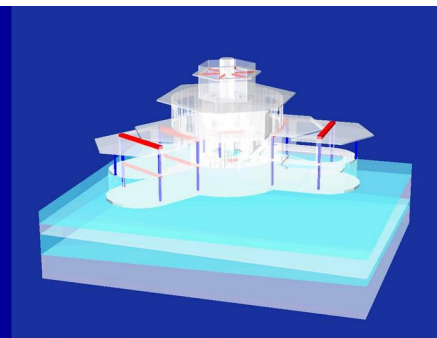
цветовое изображение изгибающих моментов в расчётных схемах перекрытий подвала и первого этажа
