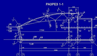
СХЕМА МЕТАЛЛОКОНСТРУКЦИЙ ПОКРЫТИЯ
