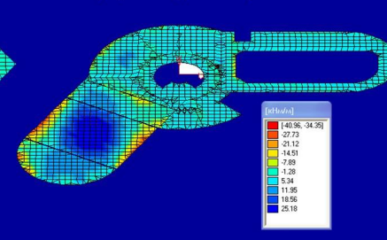
цветовое изображение изгибающих моментов в расчётных схемах перекрытий подвала и первого этажа
