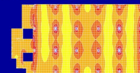
цветовое изображение моментов в расчётных схемах фундаментной плиты и встраиваемого перекрытия
