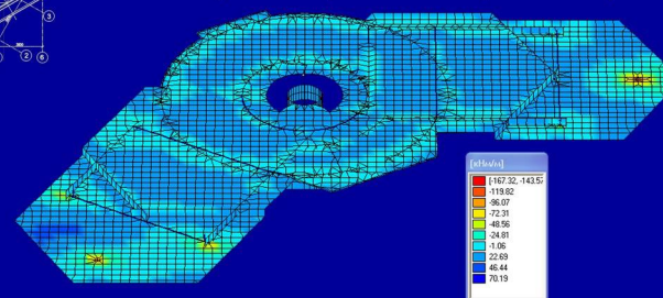
цветовое изображение изгибающих моментов в расчётных схемах перекрытий подвала и первого этажа
